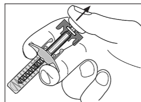
Abbildung K: Langsames Loslassen des Kolbens
